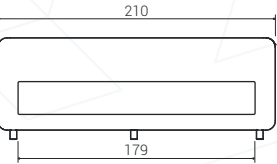
Módulo Esp. 3P + Asto. 3P
