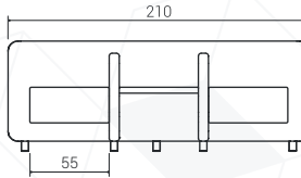
Módulo Esp. 3P + 2 Astos 1P + 2 Br centrales + Superficie
