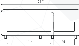
Módulo Esp. 3P + 1 Asto. 1P izq + 1 Asto. 2P izq + 1 Br central
